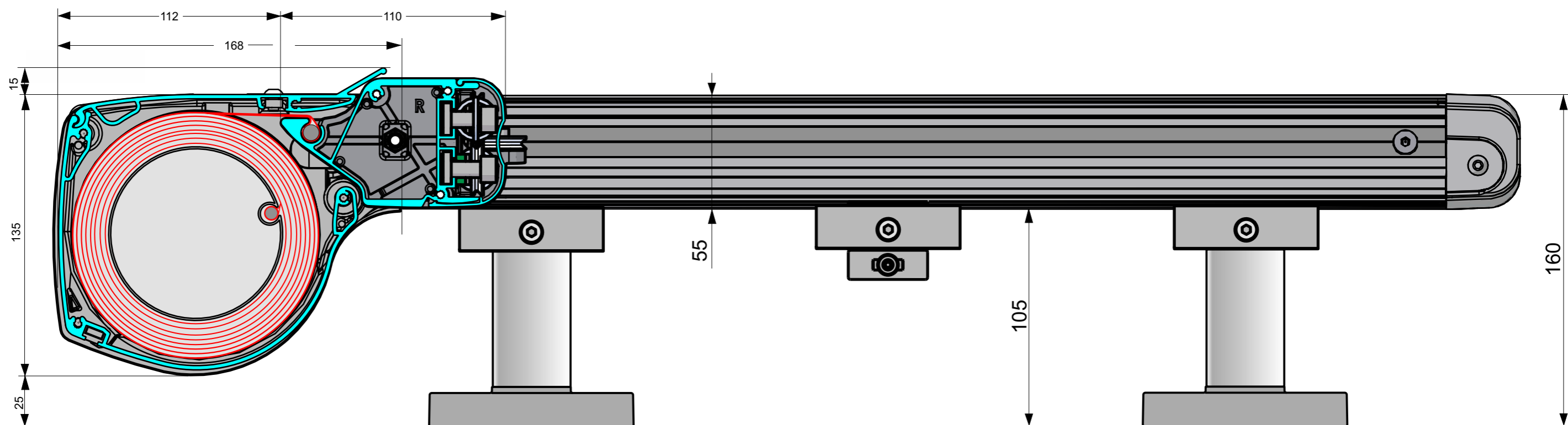
Schnitt 1 : 2
