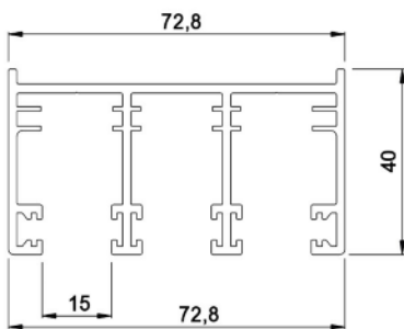
Oberschiene 3-gleisig
