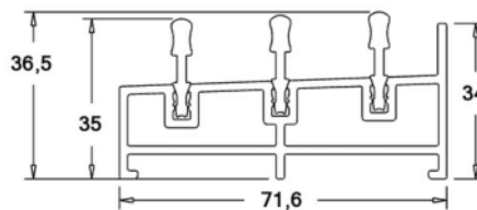
Unterschiene 3-gleisig
