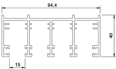
Oberschiene 4-gleisig
