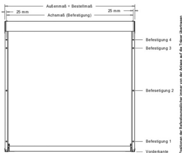
Abbildung 19: Befestigungspositionen
